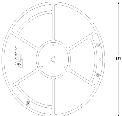
REEL DIMENSIONS
