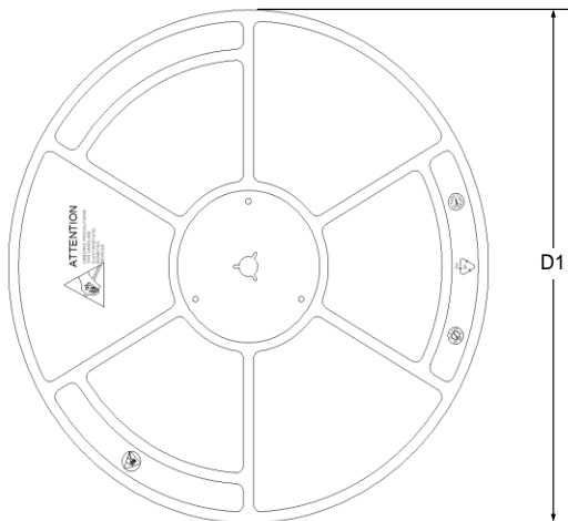
REEL DIMENSIONS
