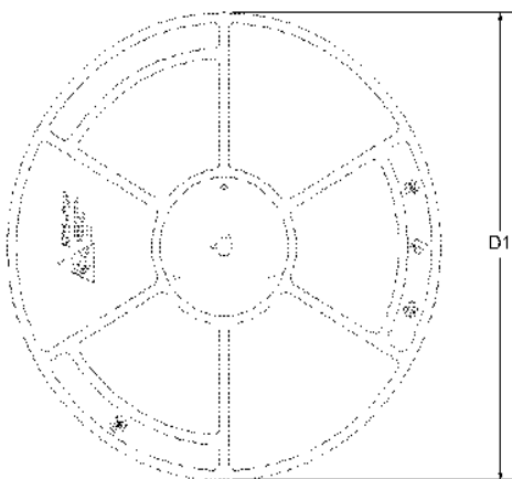
REEL DIMENSIONS
