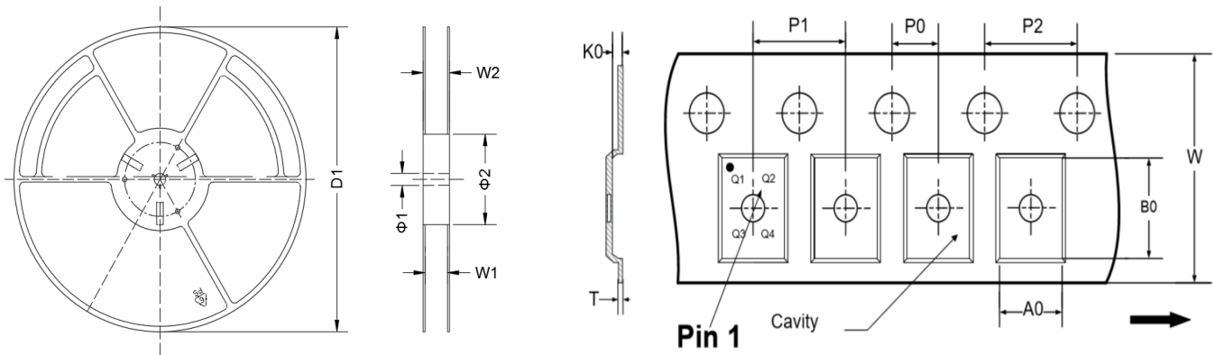
REEL DIMENSIONS
